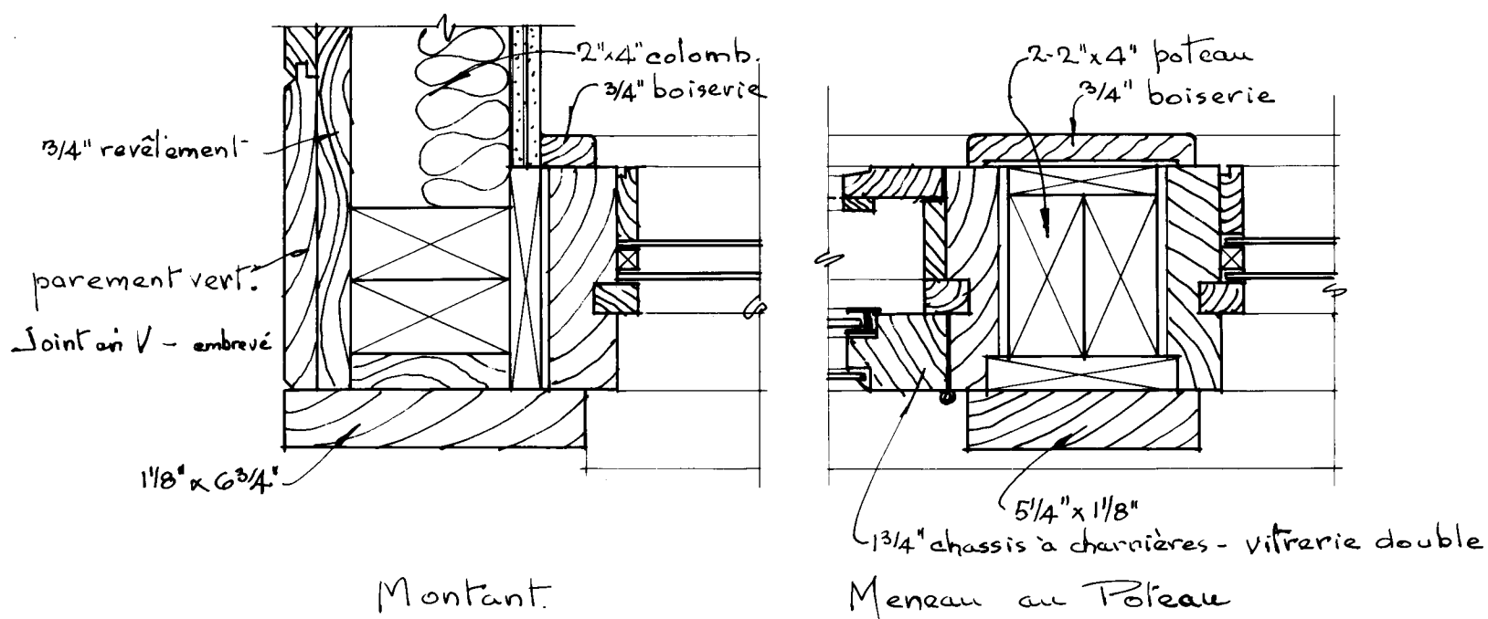
échelle : \frac{1}{4} grandeur réelle
