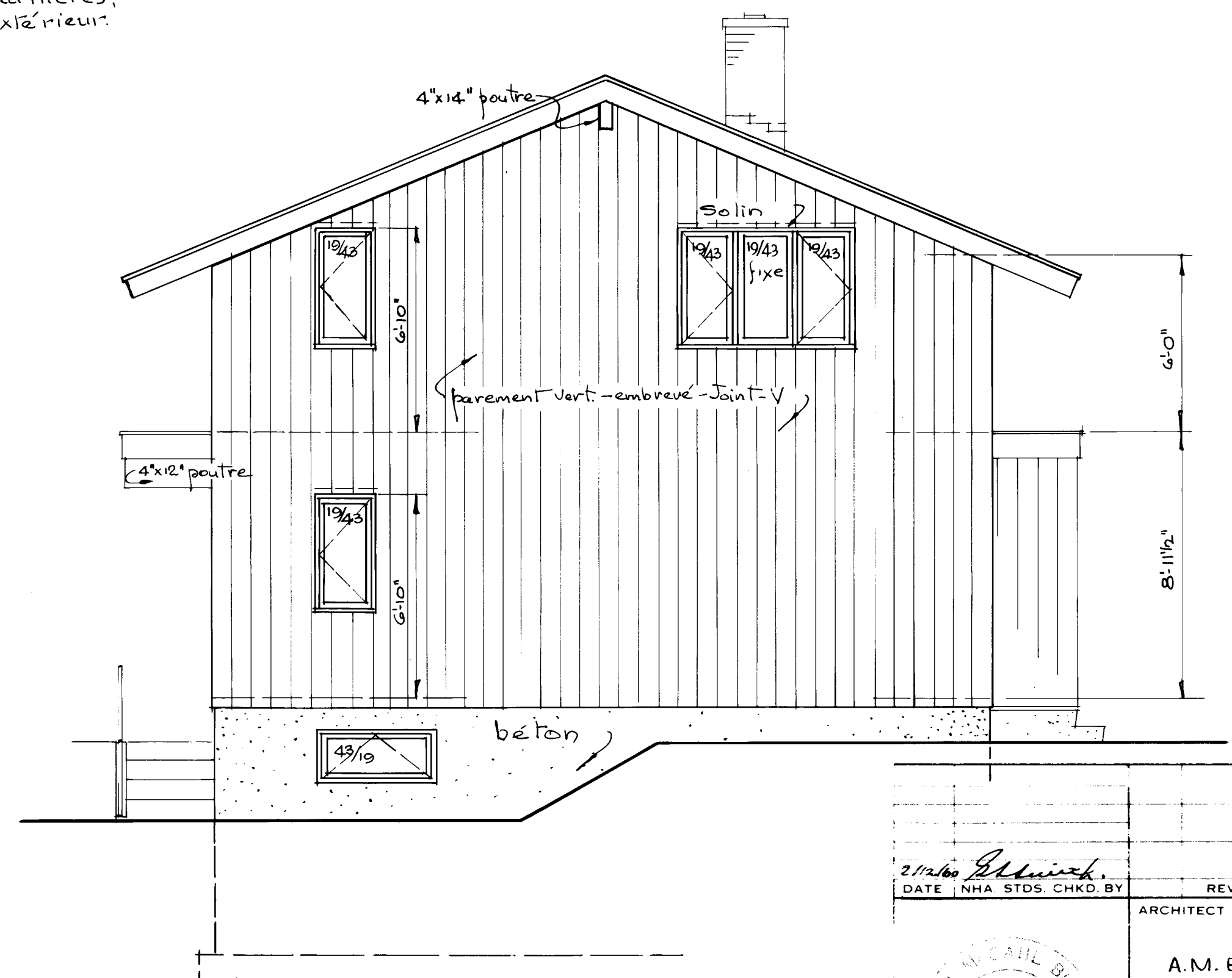
Elevation gauche échelle 1/4" = 1'-0"
