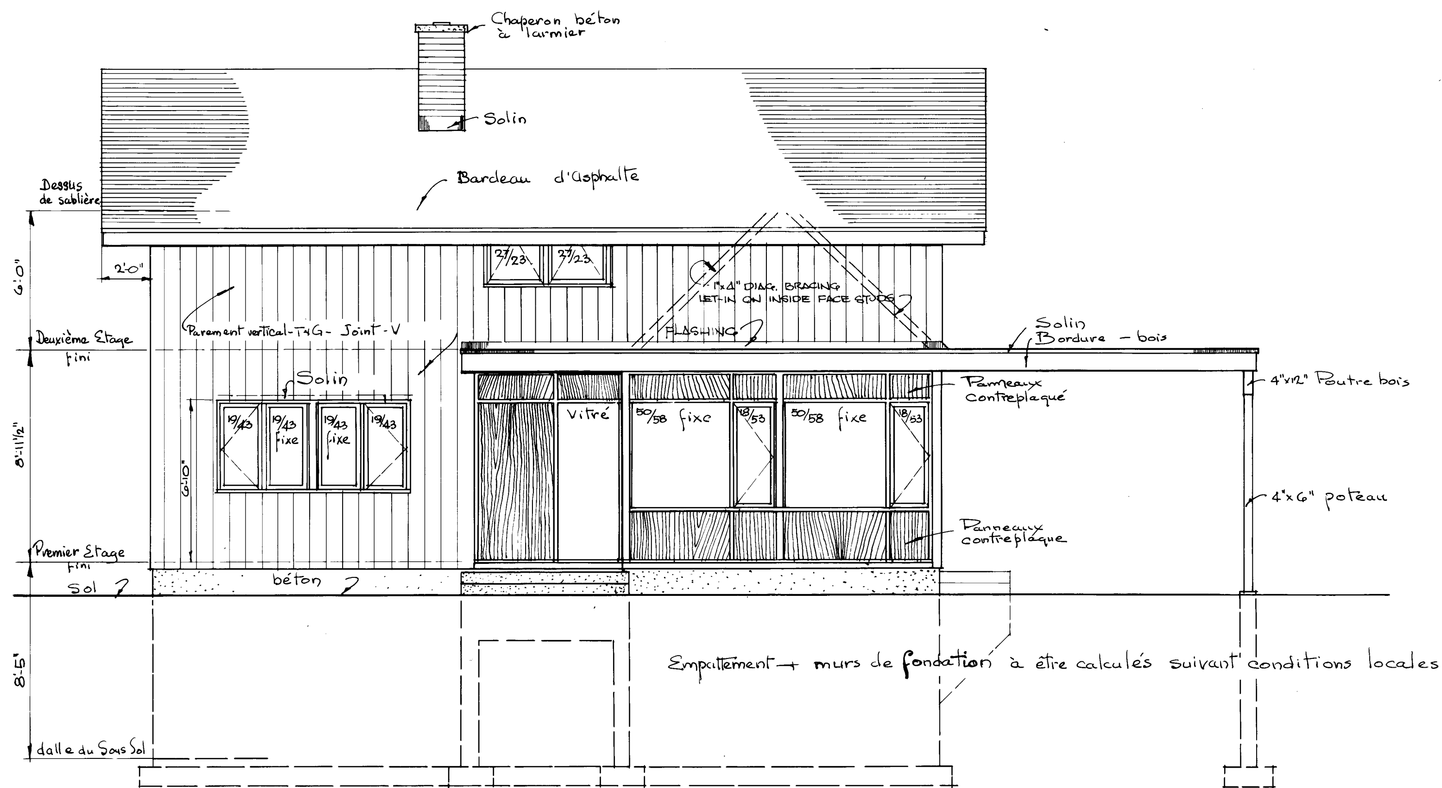
Elevation avant échelle : 1/4" = 1'-0"
