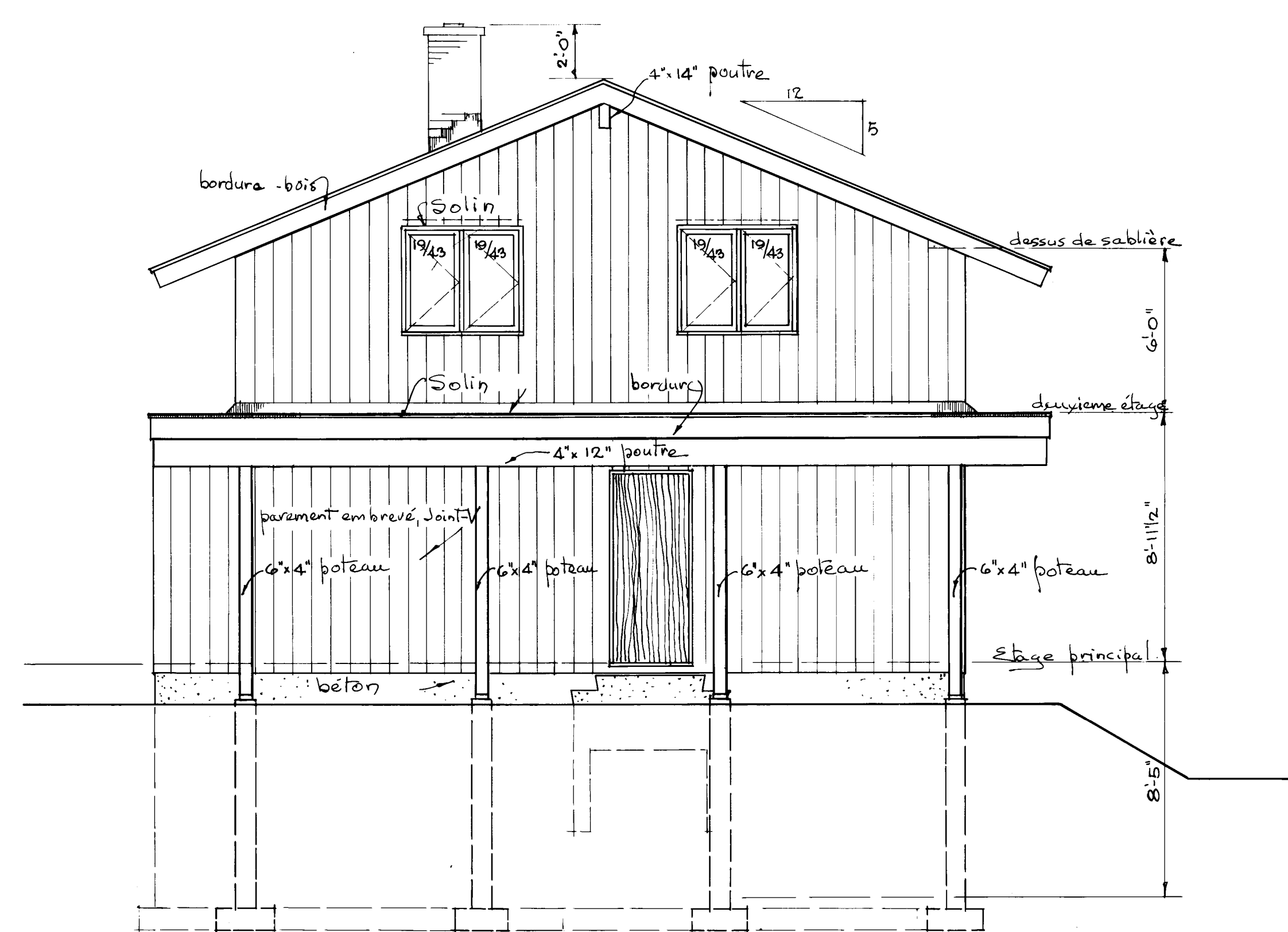
Elevation droite échelle 1/4" = 1'-0"
