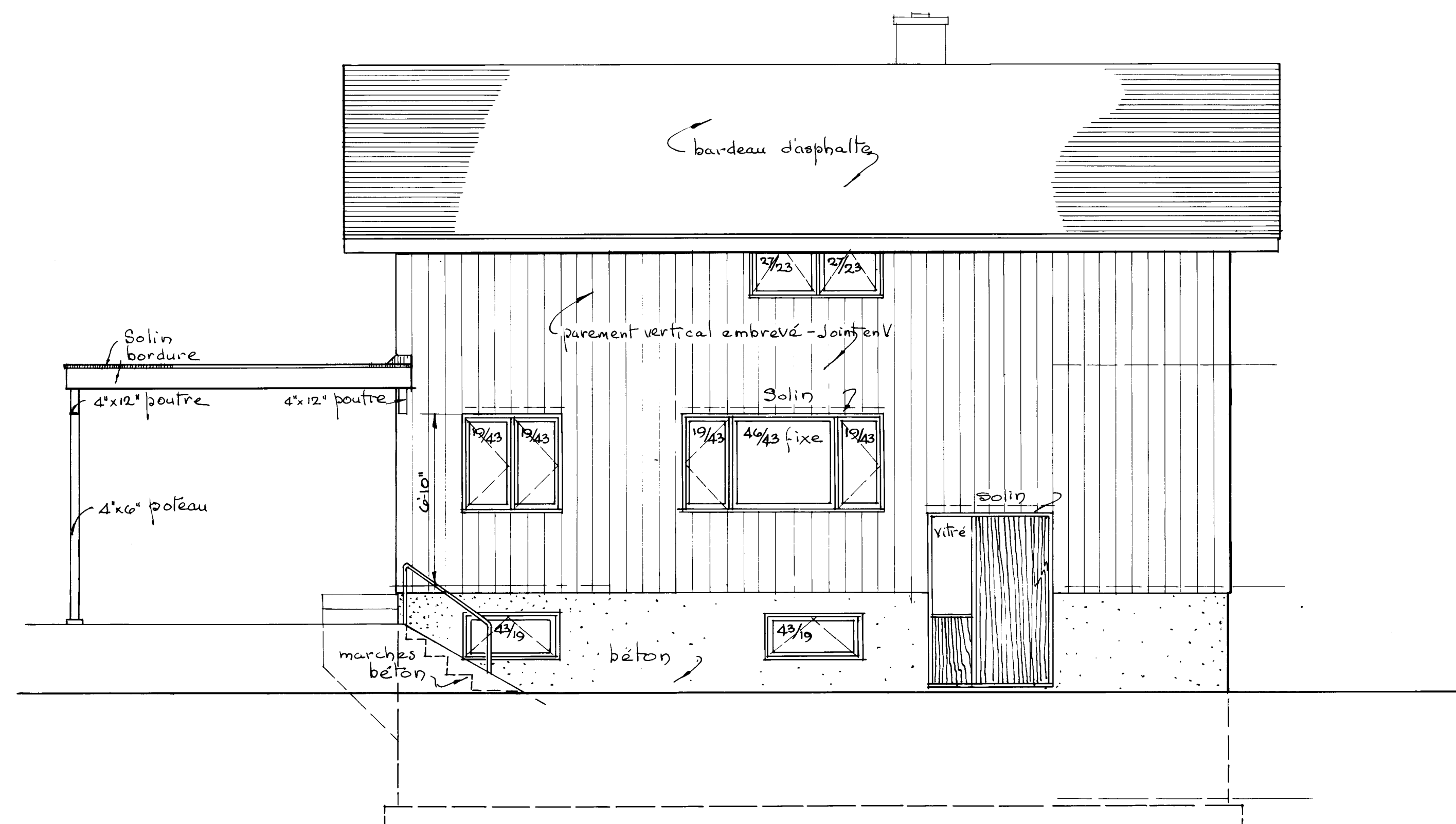
Elevation arrière échelle 1/4" = 1'-0"
