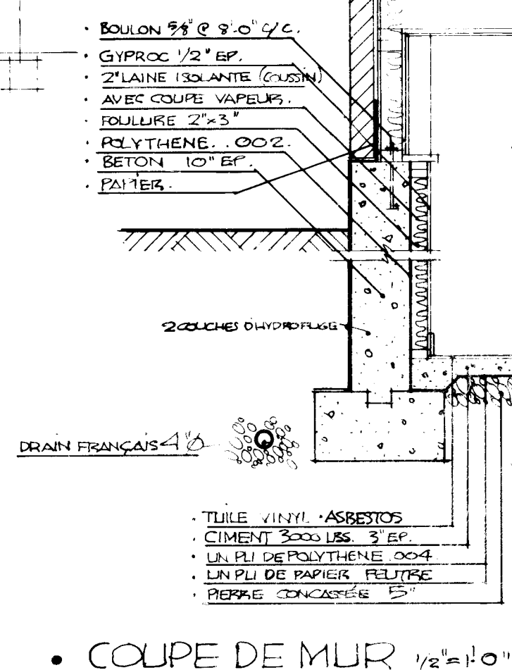
• COUPE DE MUR 1/2\"/>
