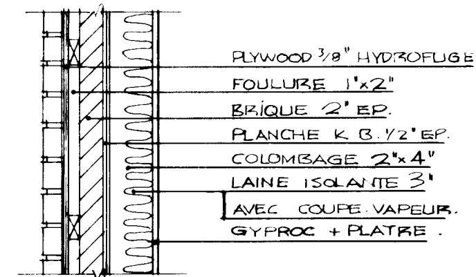
• DÉTAIL DU MUR AVEC PLYWOOD. 1" = 1'-0"
