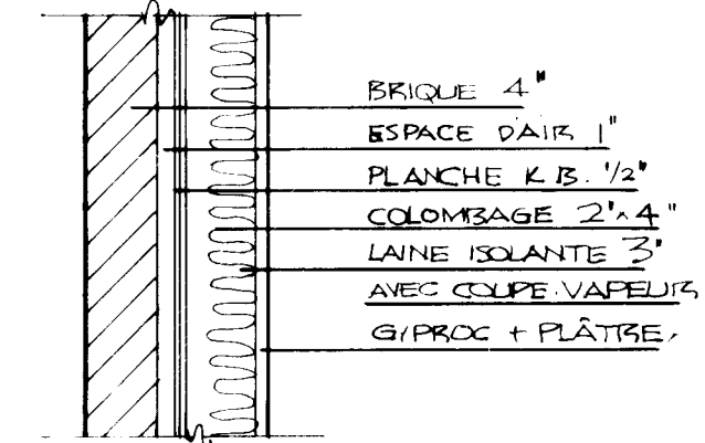
• DÉTAIL DU MUR. 1" = 1'-0"
