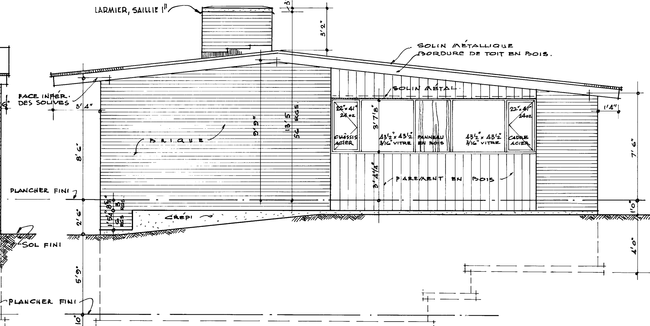
• ELEVATION GAUCHE . ÉCHELLE \frac{1}{4}'' = 1'0'' .
