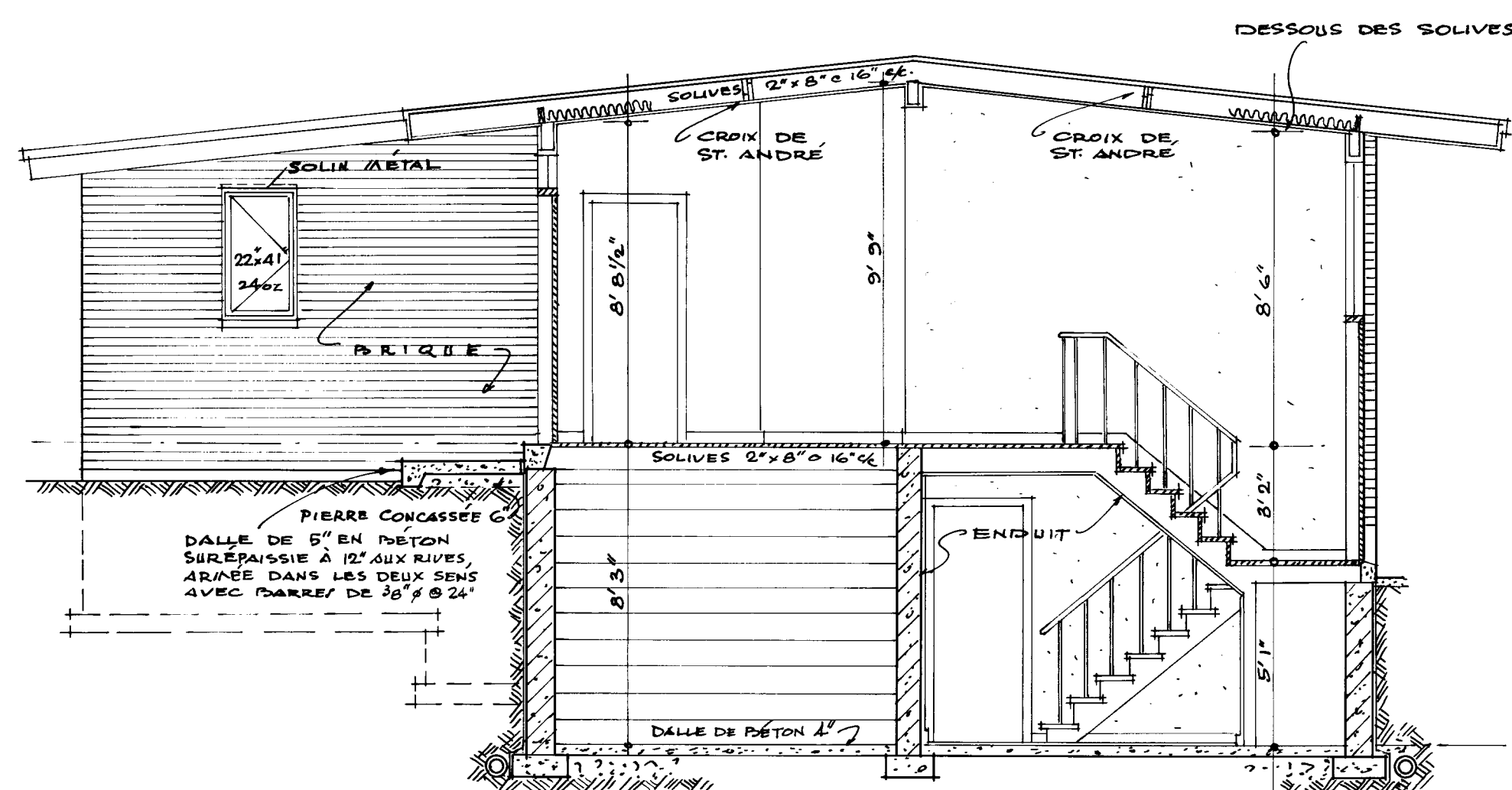
• SECTION 'B-B' • ÉCHELLE 1/4" = 1'0"
