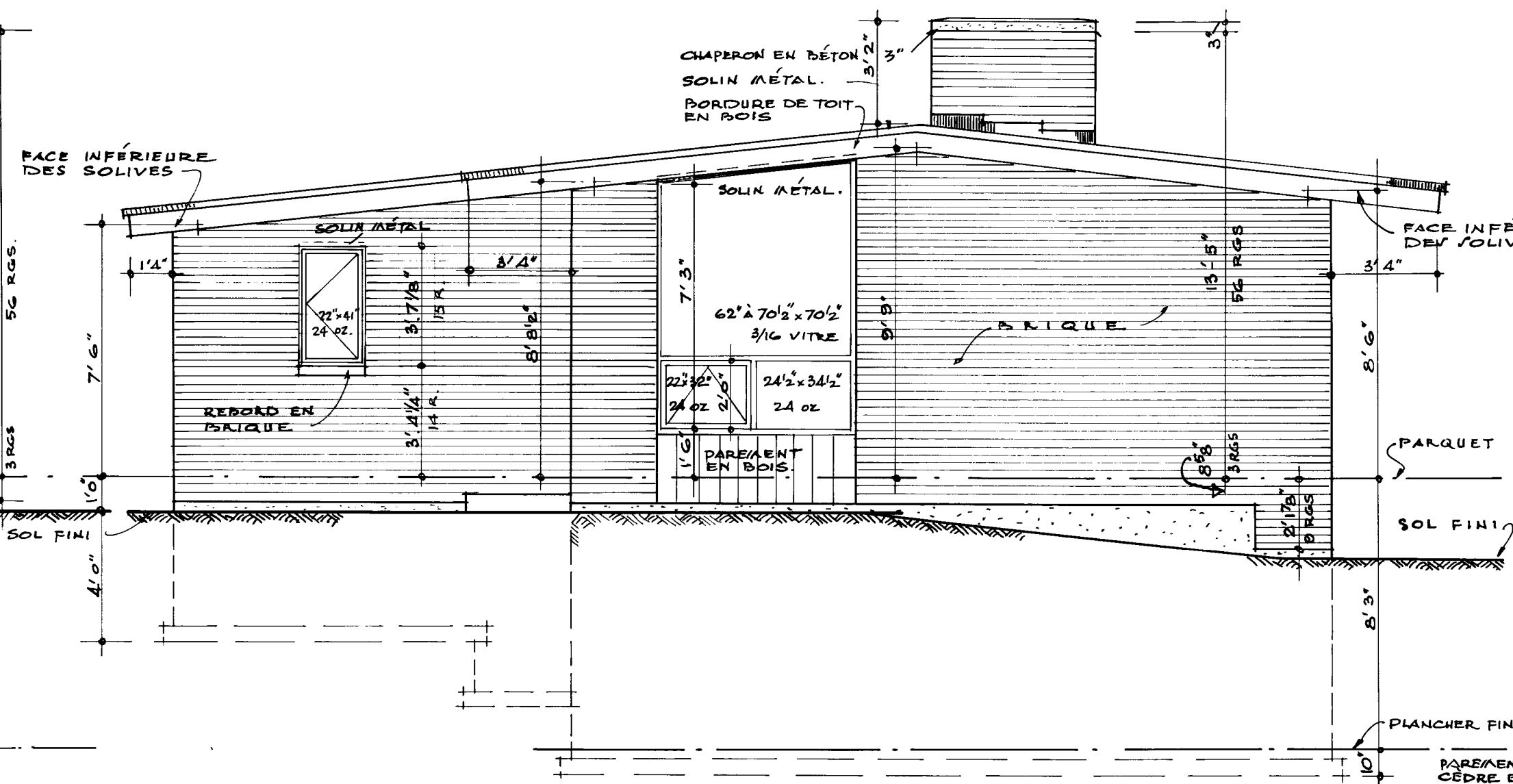
• ÉLEVATION DROITE • ÉCHELLE 1/4"=1'0"
