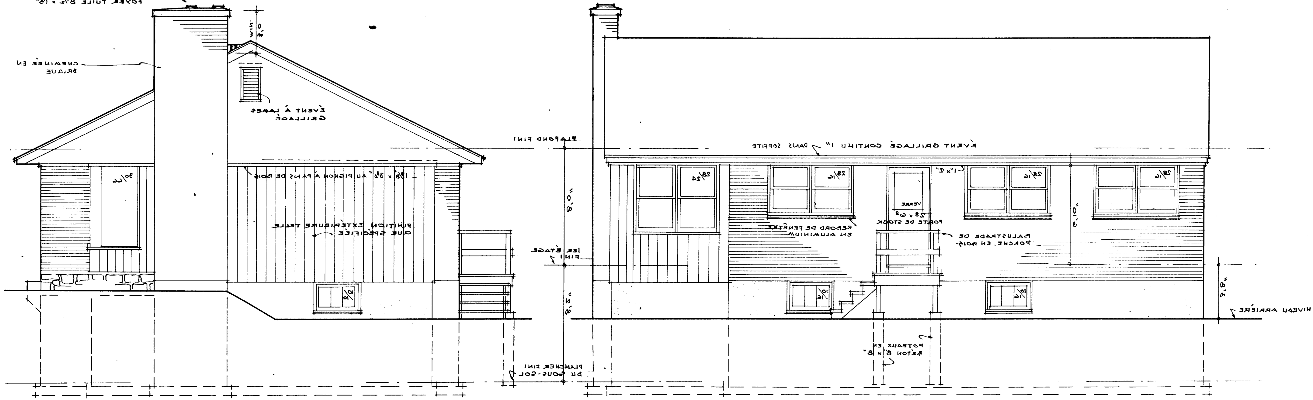
• ÉLEVATION GAUCHE • ÉCHELLE 1/8" = 1'-0"
