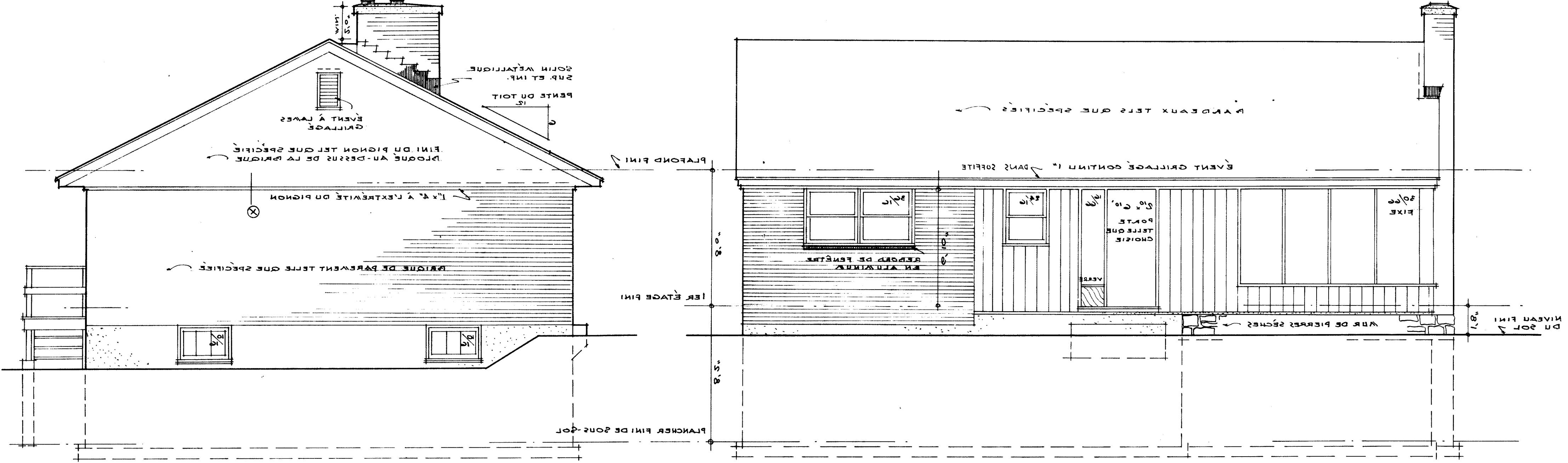
• ÉLEVATION AVANT • ÉCHELLE 1/8" = 1'-0"
