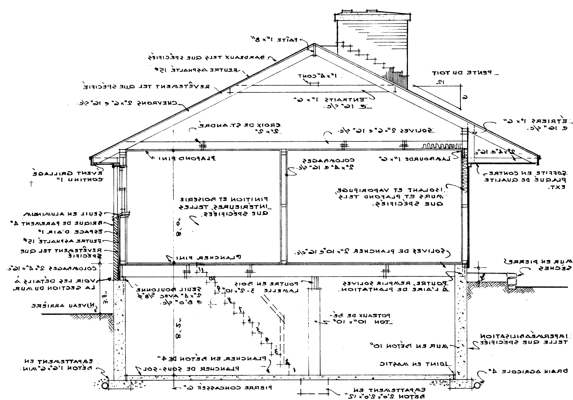
• SECTION 'A-A' •
