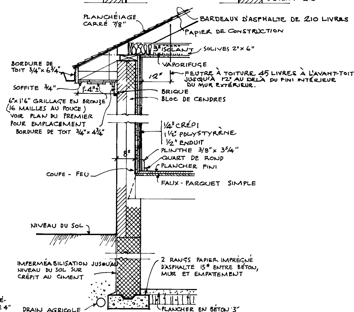
DÉTAIL DE L'AVANT-TOIT, DU MUR ET DE LA FONDATION.
