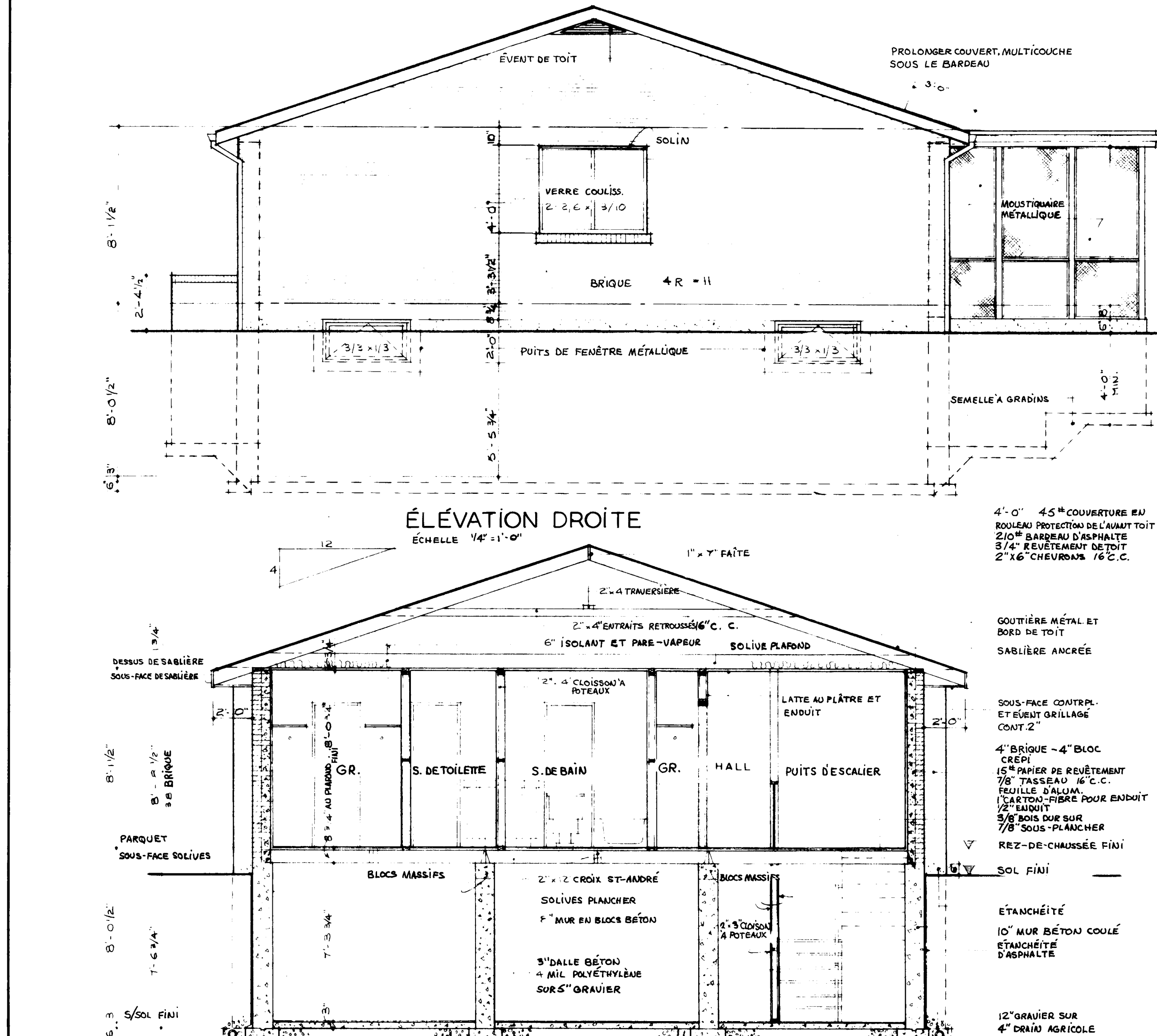
SECTION A-A ÉCHELLE 1/4" = 1'-0"
