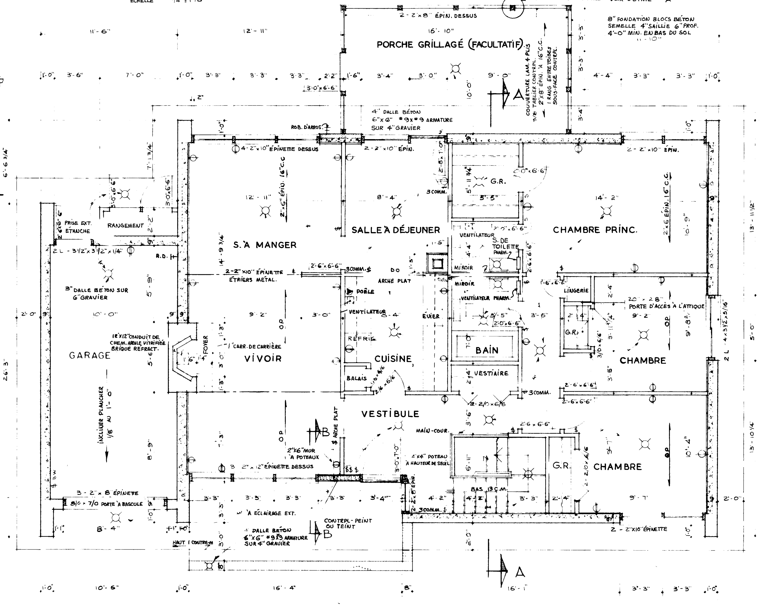
PLAN REZ-DE-CHAUSSEE ÉCHELLE 1/4" = 1'-0"
