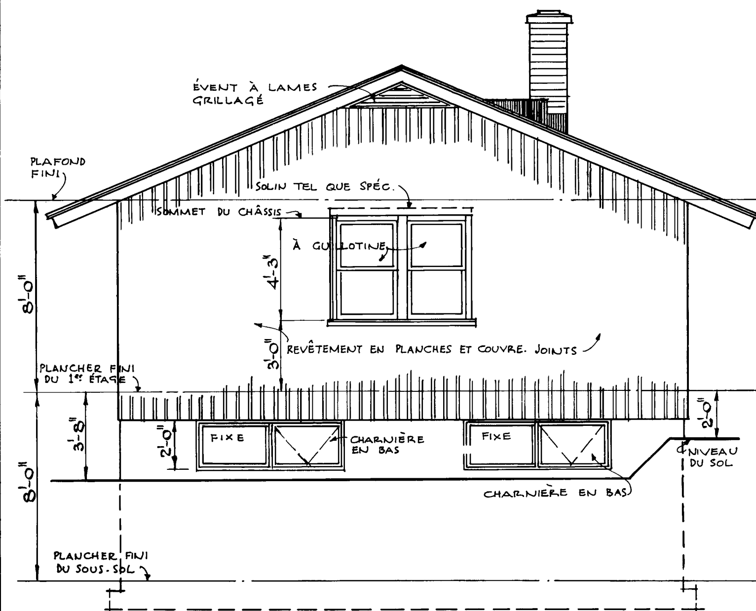
ÉLEVATION DE CÔTÉ.
