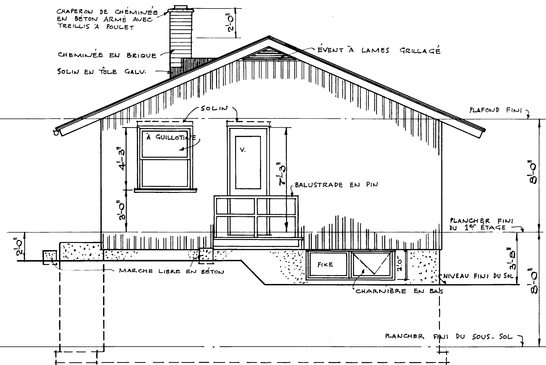
ÉLEVATION DE CÔTÉ.
